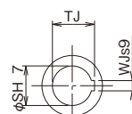
出力軸
