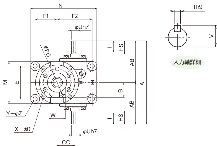
標準寸法
