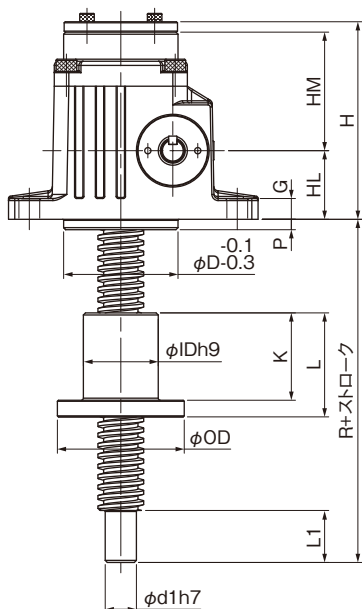
D (引上型)
