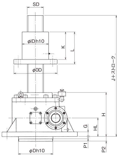
U (押し型)
