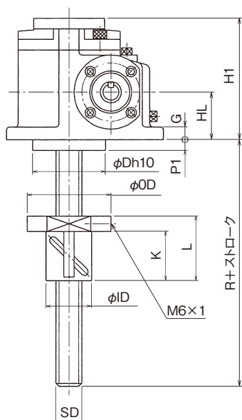
D (引上型)
