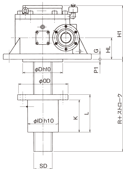
D (引上型)
