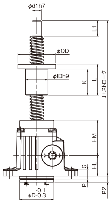
U (押し型)
