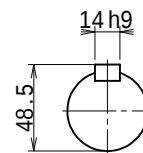
出力軸 (尺度 1/3)
