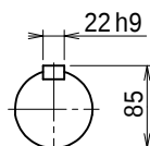
出力軸
