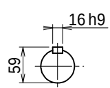
入力軸
