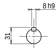
出力軸 尺度 1 / 3
