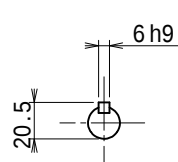
入力軸 尺度 1 / 3
