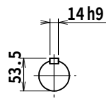
入力軸
