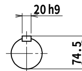
出力軸
