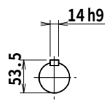
入力軸
