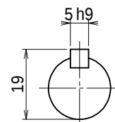
出力軸 (尺度:1/1)
