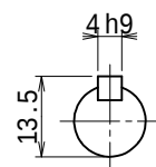
入力軸 (尺度:1/1)
