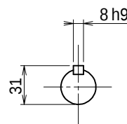
出力軸 尺度 1 / 3
