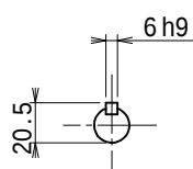
入力軸 尺度 1 / 3
