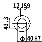
中空出力軸 (尺度 1/6)
