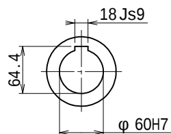
出力軸 (尺度 1/5)
