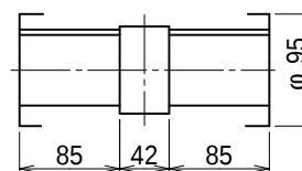
出力軸内部詳細 (尺度 1/5)
