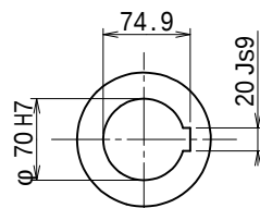
出力軸
