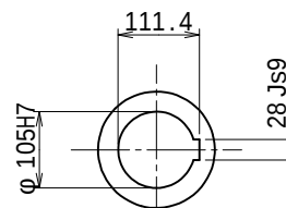
出力軸
