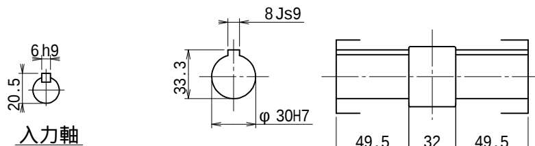
出力軸内部詳細
