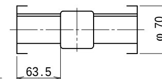
出力軸内部詳細 (尺度1/4)
