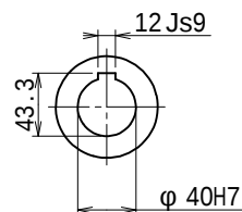
中空出力軸 (尺度1/4)
