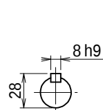
入力軸 (尺度1/3)
