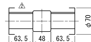
出力軸中空軸詳細 (尺度1/4)
