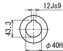
出力軸 (尺度1/4)
