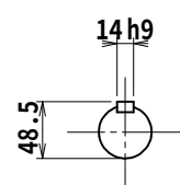
入力軸
