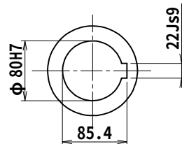
出力軸
