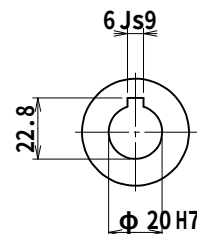
出力軸
