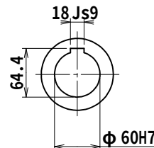
出力軸 (尺度 1/5)
