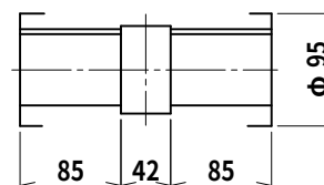
出力軸内部詳細
