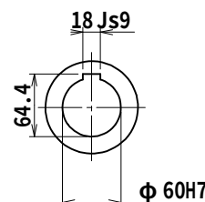
出力軸
