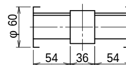
出力軸内部詳細 (尺度 1/4)
