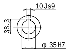
出力軸 (尺度 1/4)
