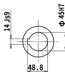
出力軸内部詳細
