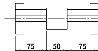
出力軸内部詳細
