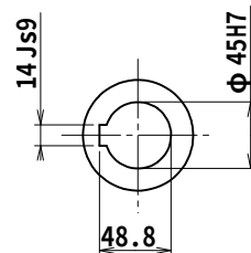
出力軸
