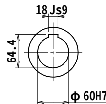
出力軸 (尺度 1/5)
