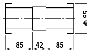
出力軸内部詳細 (尺度 1/5)
