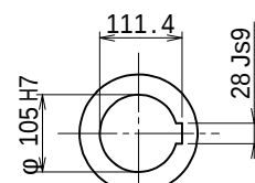
出力軸
