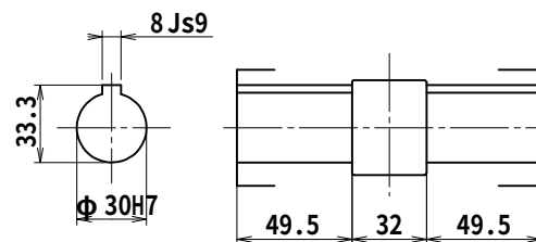
出力軸内部詳細
