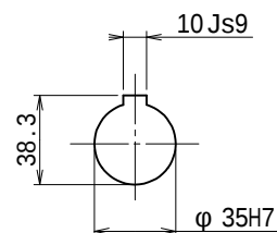
出力軸内部詳細
