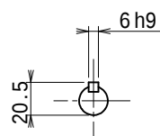
入力軸 尺度 1 / 3
