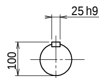
出力軸
