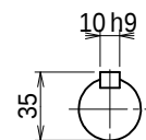
出力軸 (尺度 1/3)
