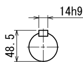
出力軸 (尺度 1/4)
