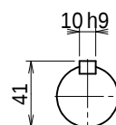
出力軸 (S=1/3)
