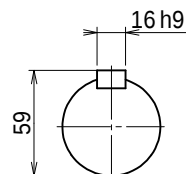
出力軸 (尺度 1/3)
