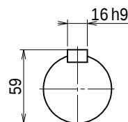
出力軸 (尺度 1/3)
