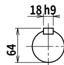
出力軸
