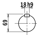
出力軸 (S=1/5)
