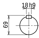
出力軸 (S=1/5)
