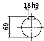
出力軸 (S=1/5)
