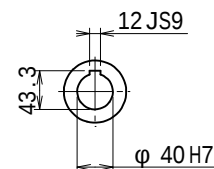
中空出力軸 (尺度 1/6)
