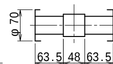
出力軸内部詳細 (尺度 1/6)
