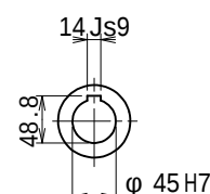
出力軸 (尺度 1/6)
