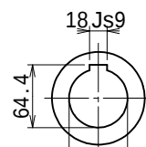
出力軸 (尺度 1/5)
