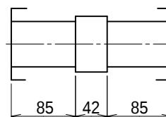
出力軸内部詳細 (尺度 1/5)
