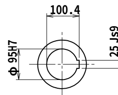
出力軸
