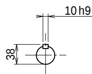
出力軸
