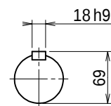
出力軸
