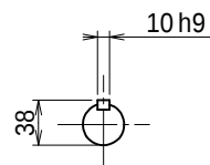
出力軸 (S=1/5)
