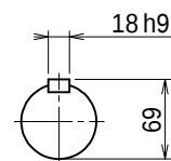
出力軸 (S=1/5)
