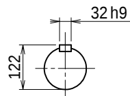
出力軸
