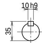
出力軸
