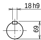
出力軸
