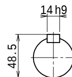
出力軸 (S=1/3)
