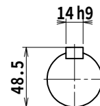
出力軸 (S=1/3)
