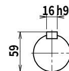
出力軸 (尺度 1/4)
